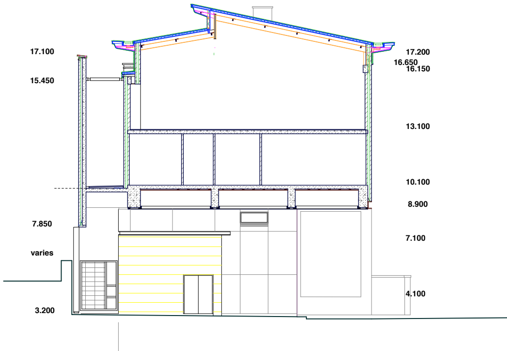
Section E3-E3
